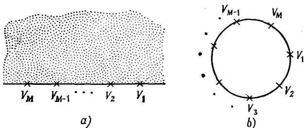
Рис. 7.7. Бесконечную полосу рис. 7.6 можно конформно отобразить на верхнюю полуплоскость, рис. a), или на единичный круг, рис. b).
