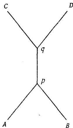
Рис. 1.5. Типичная фейнмановская диаграмма в квантовой теории поля. Четыре внешние частицы, появляющиеся в пространственно-временных точках A , B , C и D , участвуют в процессе рассеяния на уровне древесных диаграмм, взаимодействия происходят в точках p и q .
