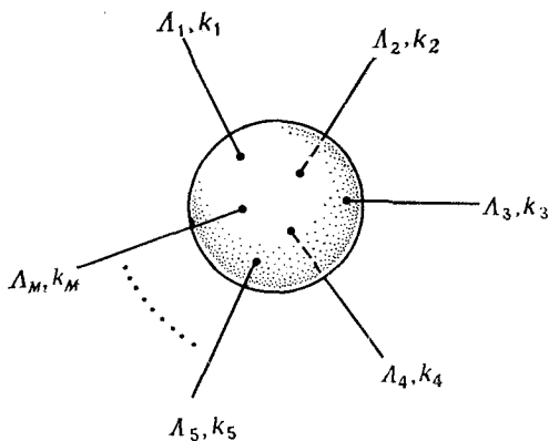
Рис. 1.12. Представление амплитуды рассеяния M внешних частиц типа \Lambda_1, \Lambda_2, \dots, \Lambda_M с импульсами k_1, k_2, \dots, k_M .
