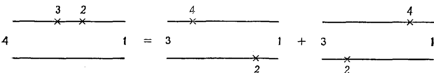
Рис. 7.9. Тождество с оператором твиста для четырехточечной амплитуды. Из рисунка видно, что когда частицы испускаются из противоположных краев мировой поверхности, то два разных способа упорядочения по времени вершинных операторов отвечают одному и тому же циклическому упорядочению всех четырех частиц.
