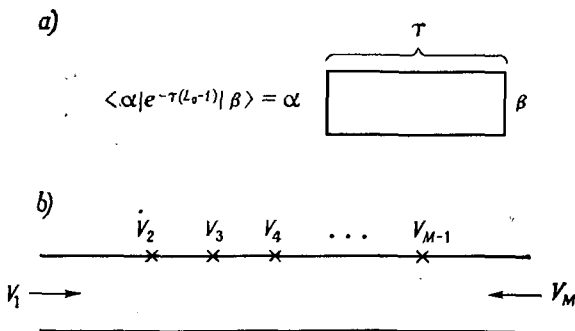
Рис. 7.6. Пропагатор (L_0 - 1)^{-1} = \int d\tau e^{-\tau(L_0-1)} описывает распространение струны на расстояние \tau в мнимом времени и тем самым порождает полосу шириной \pi и длиной \tau , рис. a). Дерево же \langle 1 | V_2(L_0 - 1)^{-1} V_3 \dots V_{M-1} M \rangle представляется тогда в виде интеграла по бесконечной полосе, где полубесконечные куски слева и справа соответствуют начальному и конечному состояниям |M\rangle и |1\rangle , рис. b).
