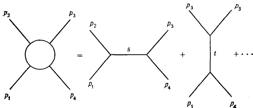
Рис. 1.1. Упругий процесс рассеяния с налетающими частицами с импульсами p_1 , p_2 и уходящими частицами с импульсами p_3 , p_4 (мы условимся помечать буквами входящие импульсы.) Приведены диаграммы и в s -, и в t -каналах. В теории поля амплитуда строится как сумма выражений, соответствующих диаграммам в каналах s и t .
