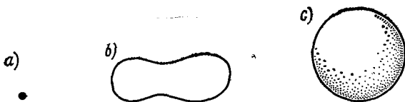
Рис. 2.1. Теорию точечной частицы (a) можно обобщить на случай струны (b) или мембраны (c).
