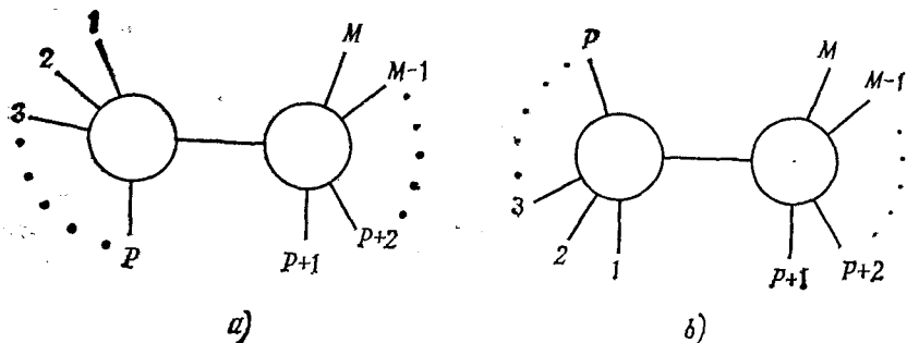
Рис. 6.2. У примитивной амплитуды A(1, \dots, M) есть полюс по инвариантной переменной S = -(k_1 + k_2 + \dots + k_p)^2 , вычет в котором представим в виде произведения двух других примитивных амплитуд, как это представлено на рис. а). Другая примитивная амплитуда, но имеющая полюс с таким же вычетом, изображена на рис. б).
