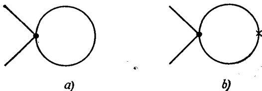
Рис. 3.7. Однопетлевой контрчлен в нелинейной сигма-модели появляется из диаграммы, изображенной на рис. а). При проверке вейлевской инвариантности в описанном формализме мы встречаемся еще и с диаграммой, изображенной на рис. б), где крестик обозначает вставку кинетического члена с коэффициентом \varepsilon\Phi .
