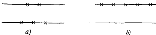
Рис. 7.11. Испускание бозонов из фермионной струны, рис. a ); на рис. b ) все бозоны испускаются из одного и того же края мировой поверхности.
