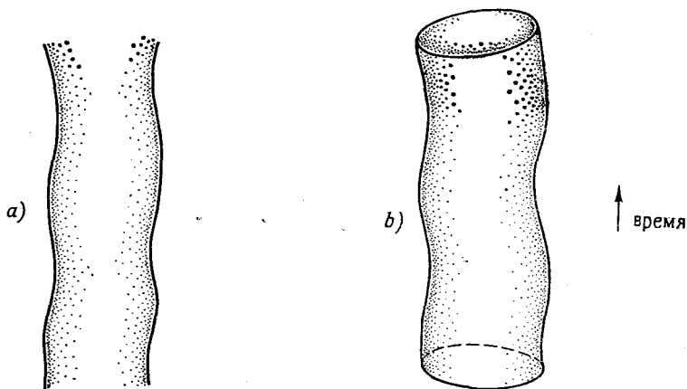
Рис. 1.3. Открытая (а) или замкнутая (б) струна, распространяясь в пространстве Минковского, замечает двумерную поверхность, известную как мировая поверхность струны. Из классических уравнений свободной теории струн следует, что эта поверхность должна быть минимальной, т.е. обладать наименьшей площадью.
