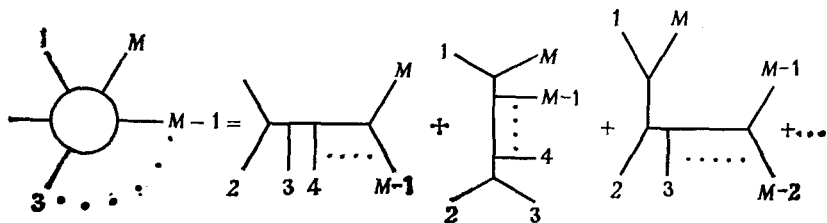
Рис. 7.4. В теории поля древесная амплитуда для M частиц 1, 2, 3, \dots, M представляется в виде суммы целого набора фейнмановских диаграмм, отвечающих полюсам в различных частных каналах.
