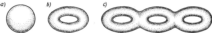
Рис. 3.2. Диаграммы мировой поверхности в теории замкнутых ориентированных струн: (а) древесная, (б) однопетлевая, (с) многопетлевая.
