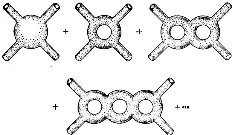
Рис. 1.8. Здесь мы схематически изобраили все диаграммы замкнутой струны, которые дают вклад в четырехчастичную амплитуду; в каждом порядке теории возмущений имеется одна и только одна диаграмма.
