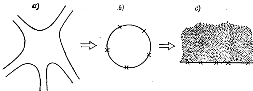
Рис. 1.15. На рис. a схематически изображена «планарная» мировая поверхность, соответствующая рассеянию открытых струн. Она может быть конформно отображена на диск (рис. b ) или на верхнюю полуплоскость комплексной плоскости (рис. c ). В любом из этих случаев внешние состояния открытых струн появляются как вставки на границе; на рис. b и c они обозначены \otimes .
