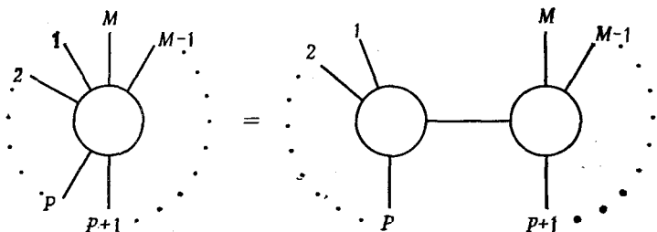
Рис. 7.3. Из условия древетной унитарности вытекает, что M -частичная амплитуда для набора 1, 2, 3, \dots, M в канале 1, 2, 3, \dots, P \rightarrow P+1, \dots, M должна иметь вычет, представимый в виде произведения древетных амплитуд для наборов 1, 2, 3, \dots, P и P+1, \dots, M .
