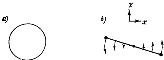
Рис. 2.3. На рис. a схематически изображена замкнутая струна радиуса R , находящаяся в начальный момент в состоянии покоя. На рис. b показана открытая струна, закручивающаяся в плоскости x-y .
