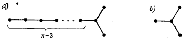
Рис. 5.1. а) — схема Дынкина для группы SO(2n) ; б) — схема Дынкина для группы SO(8) симметрична относительно перестановок трех внешних линий.
