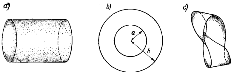
Рис. 3.6. Наипростейшей однопетлевой мировой поверхностью открытой струны является цилиндр (рис. а). Его всегда можно конформно отобразить на стандартное кольцо в комплексной плоскости, как показано на рис. б. Другой однопетлевой мировой поверхностью струны является перекрученный цилиндр, или лента Мёбиуса (рис. с), которую можно рассмотреть аналогично.
