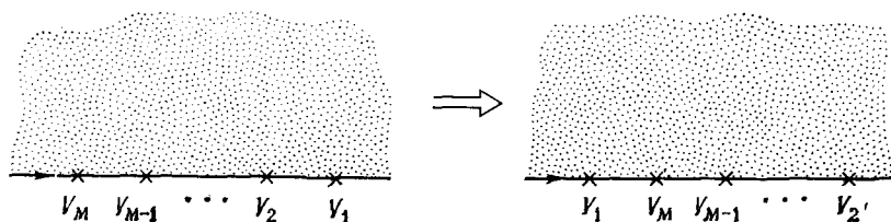
Рис. 7.8. Преобразование SL(2, R) может превратить вершинный оператор, стоящий «последним» в цепочке из M вертеков, в «первый».
