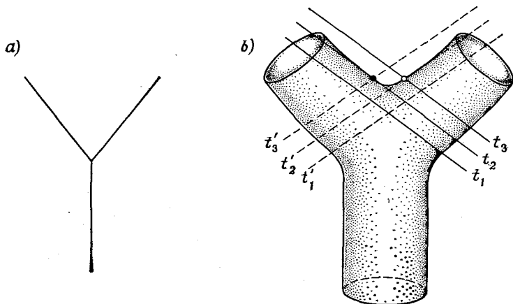
Рис. 1.6. Вершины взаимодействия в теории поля и в теории струн: на рис. a точечная частица расщепляется на две; на рис. b замкнутая струна расщепляется на две. На рис. b поверхности постоянного времени в двух различных лоренцевых системах отсчета 1 и 2 изображены сплошной и штриховой линиями соответственно.
