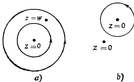
Рис. 6.5. Контуры z -интегрирования для A_k A_{k'} и A_{k'} A_k выбираются так, чтобы точка w лежала соответственно вовне или внутри контура, рис. a ). Таким образом, разности отвечает контур вокруг единственной потенциально сингулярной точки z = w , рис. b ).
