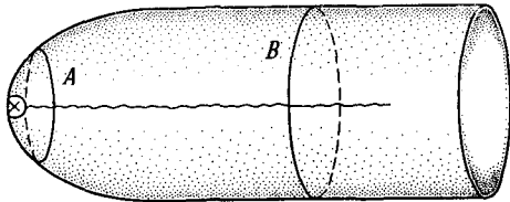
Рис. 7.13. Цель этого рисунка — прояснить сущность состояния, порождаемого фермионным вершинным оператором; место вставки этого оператора обозначено меткой \otimes .
