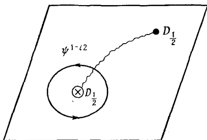
Рис. 7.14. Корреляционная функция \langle D_{1/2}, D_{1/2}, \psi^{1-i2} \rangle меняет знак, когда мы пронесим поле \psi^{1-i2} вдоль малого замкнутого контура, окружающего одно из D ; это значит, что D порождают разрезы для поля \psi .
