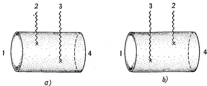
Рис. 7.10. Две диаграммы, дающие вклад в четырехчастичную древетную амплитуду для замкнутой струны. Рис. а) отвечает пропагатору в s -канале, рис. б) — пропагатору в u -канале, а их сумма дает полную кроссинг-симметричную амплитуду.
