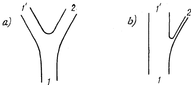
Рис. 2.4. Когда одна открытая струна расщепляется на две, как в случае а), все из них могут, вообще говоря, быть вне массовой поверхности. Если одна из струн в конечном состоянии находится на массовой поверхности, как в чае б), то она имеет ширину порядка \hbar и является в некотором смысле точечноподобной.
