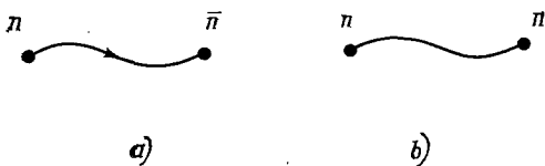
Рис. 2.5. Ориентированные и неориентированные открытые струны. Струна имеет ориентацию (рис. a ), если заряды на ее концах различны (как в КХД с обычной калибровочной группой SU(n) ), тогда как струна не имеет ориентации (рис. b ), если заряды на ее концах одинаковы, как в калибровочной теории с калибровочной группой SO(n) или Sp(n) . Для замкнутой струны понятие ориентации также является важным, хотя и более абстрактным.
