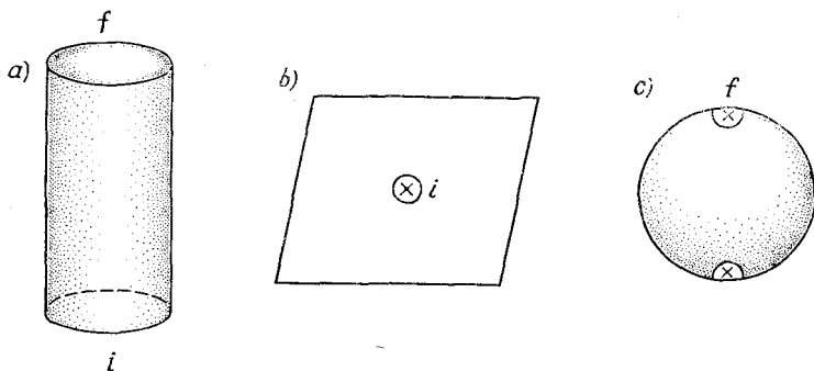
Рис. 1.11. Мировая поверхность с одной налетающей и одной уходящей струной (изображенная на рис. а) может быть описанным в тексте способом конформно отображена во многие другие фигуры. Ее можно отобразить в плоскость (рис. б), на которой налетающая струна появляется в начале координат, а уходящая струна — на бесконечности (не показано) или в сфере (рис. с), где налетающая и уходящая струны появляются в южном и северном полюсах.
