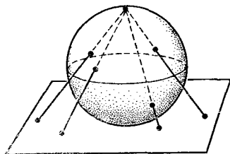
Рис. 1.13. Стереографическая проекция две-сферы S^2 на плоскость.
