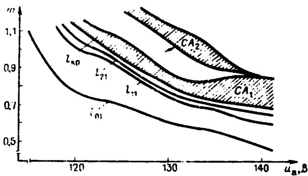
Р и с. 8.4. Экспериментальная бифуркационная диаграмма режимов колебаний на плоскости параметров m , u_a ; CA_1 и CA_2 – аттракторы 1-й и 2-й зон стохастичности. Остальные обозначения те же, что и на рис. 8.1.
