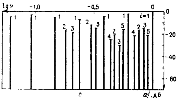
Р и с. 12.14. Экспериментальный спектр потока ( a ) и расчетный спектр отображения ( б ) вблизи критической точки разрушения тора; g = 0,3
