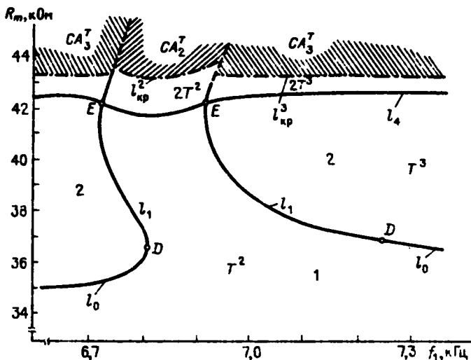
Р и с. 13.13. Бифуркационная диаграмма режимов T^2 и T^3 . Физический эксперимент для f_1 = 8,97 кГц, V_1 = 0,8 В, V_2 = 0,15 В
