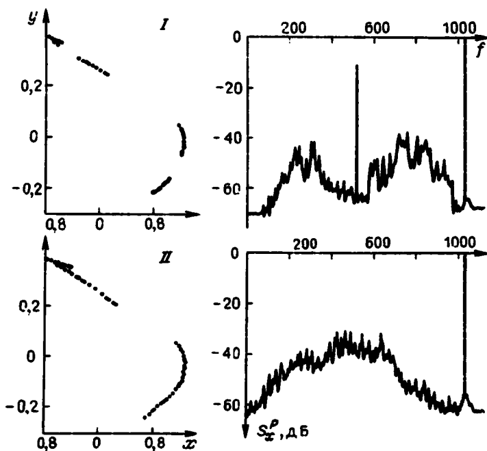
Р и с. 10.12. Фазовые портреты (слева) и спектры мощности (справа) отображения Хенона при прохождении параметром точки бифуркации связности: I - b = 0.3, a = 1.07 ; II - b = 0.3, a = 1.10
