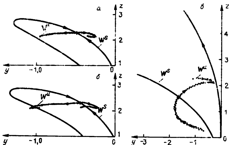
Рис. 10.10. Устойчивые и неустойчивые сепаратрисы седловых циклов системы (7.38) на секущей плоскости x = 0 : а - m = 1.09 , цикл 2\Gamma_0 ; б - m = 1.10 , цикл 2\Gamma_0 ; в - m = 1.09 , цикл \Gamma_0 .
