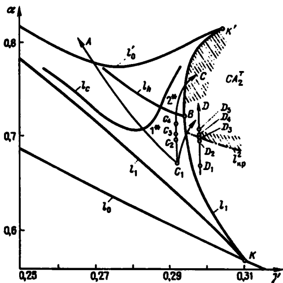
Р и с. 13.8. Бифуркационная диаграмма системы (13.7) в окрестности резонанса 2/5
