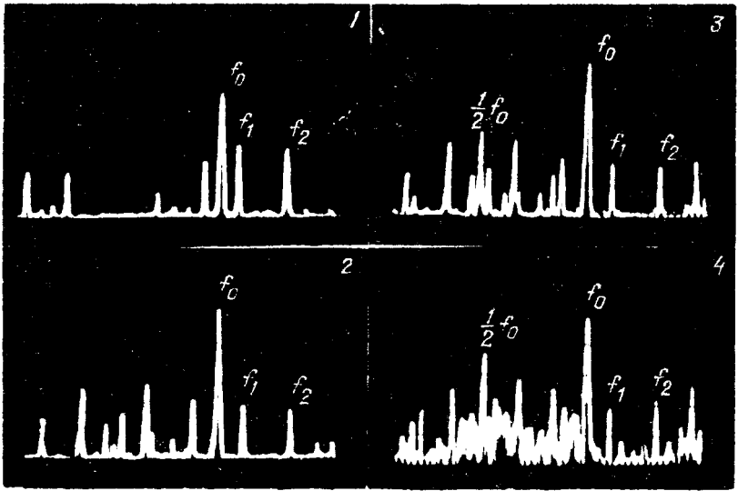
Р и с. 13.15. Переход к хаосу ( CA_1^T ), сопровождающийся бифуркацией удвоения периода трехмерного тора
