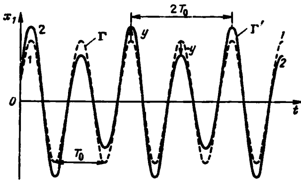
Р и с. 3.10. Бифуркация удвоения периода на примере временной зависимости фазовой координаты x_i(t) с параметром \mu < \mu^* (1) и \mu \geq \mu^* (2)
