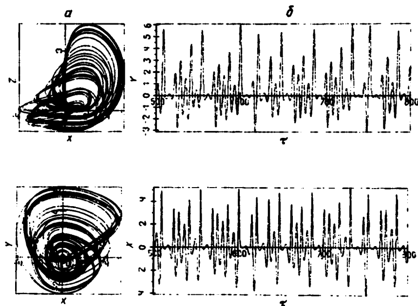
Р и с. 10.6. Двумерные проекции фазовой траектории (а) и временные зависимости y(t) , x(t) (б) хаотического аттрактора первой зоны в системе (7.38) ( m = 1,5 , g = -0,2 )
