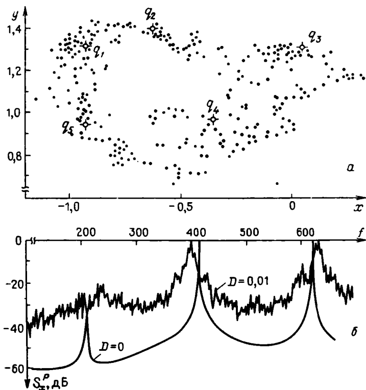
Р и с. 13.17. а – Отображение системы (13.16) на фазовой плоскости для D = 0 (точки q_1 - q_5 ) и D = 0,01 (хаотическое множество). б – Соответствующие спектры мощности процессов
