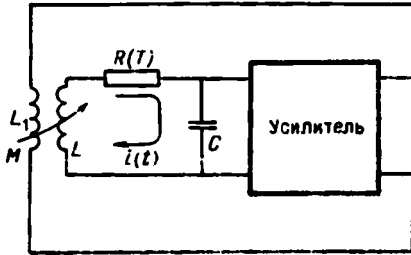
Рис. 7.3. Классическая схема генератора с инерционной нелинейностью
