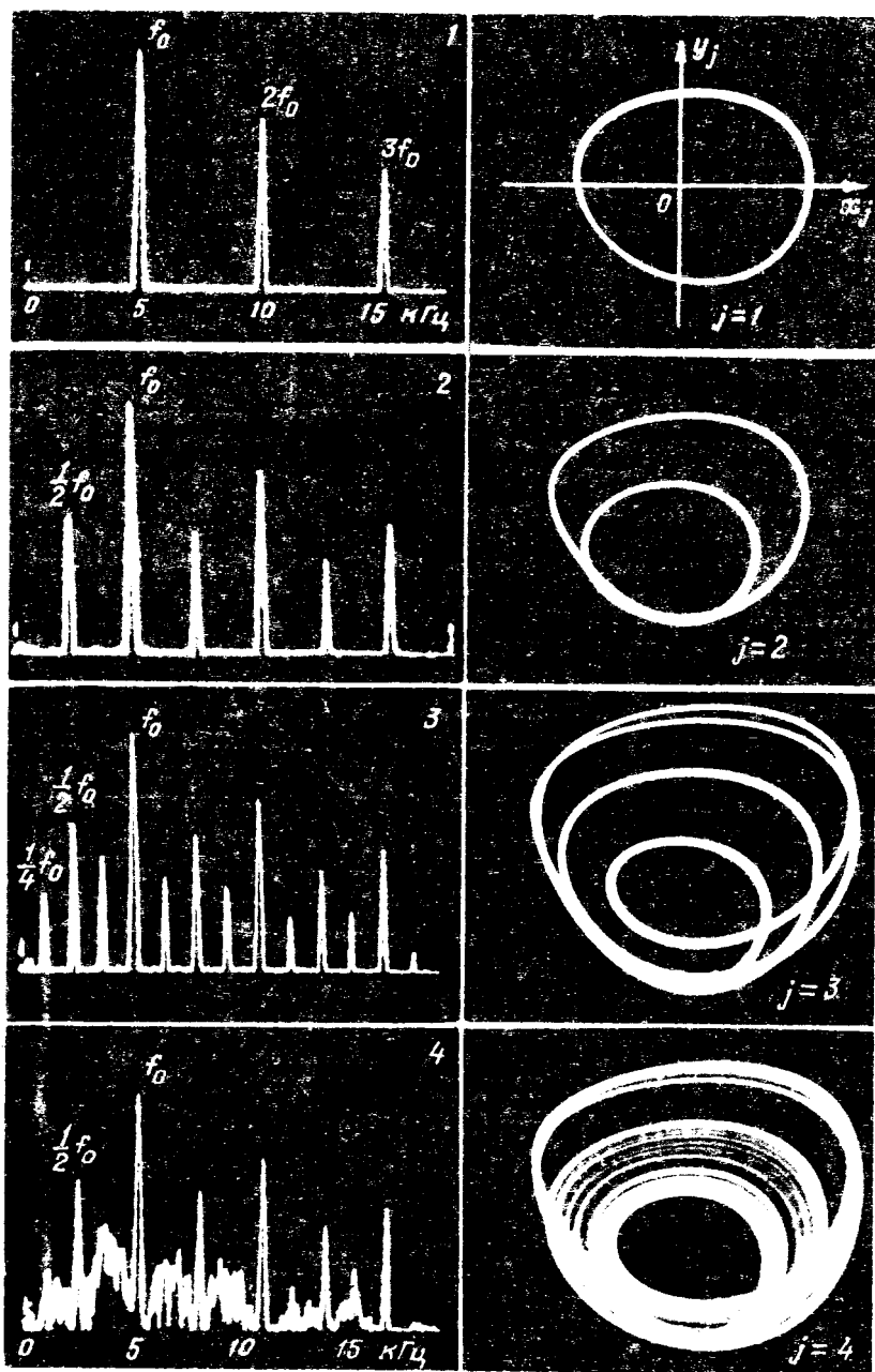
Р и с. 14.6. Эволюция спектров колебаний (слева) и проекций фазовых траекторий (справа) при движении в направлении P , диаграммы рис. 14.5
