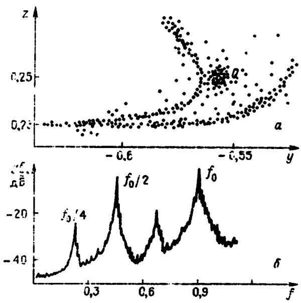
Р и с. 9.6. Сечение флуктуаций (а) и спектр мощности (б) при индуцированной мультипликативным шумом перемежаемости ( m = 1,1522, g = 0,3, D = 0,01, p = 0,01 )
