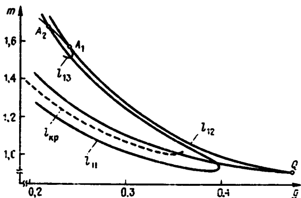
Р и с. 7.11. Бифуркационная диаграмма для семейства 2-тактных циклов \Gamma_1^i(m, g) ; l_{кр} - линия критических значений параметров, пересечению которой отвечает переход к хаосу
