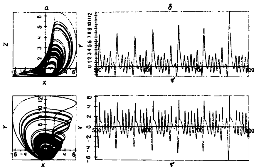
Рис. 10.4. Двумерные проекции фазовой траектории (а) и временные зависимости y(t) , x(t) (б) аттрактора Шильникова в системе (7.3к) ( m = 1.45 , g = 0.3 )
