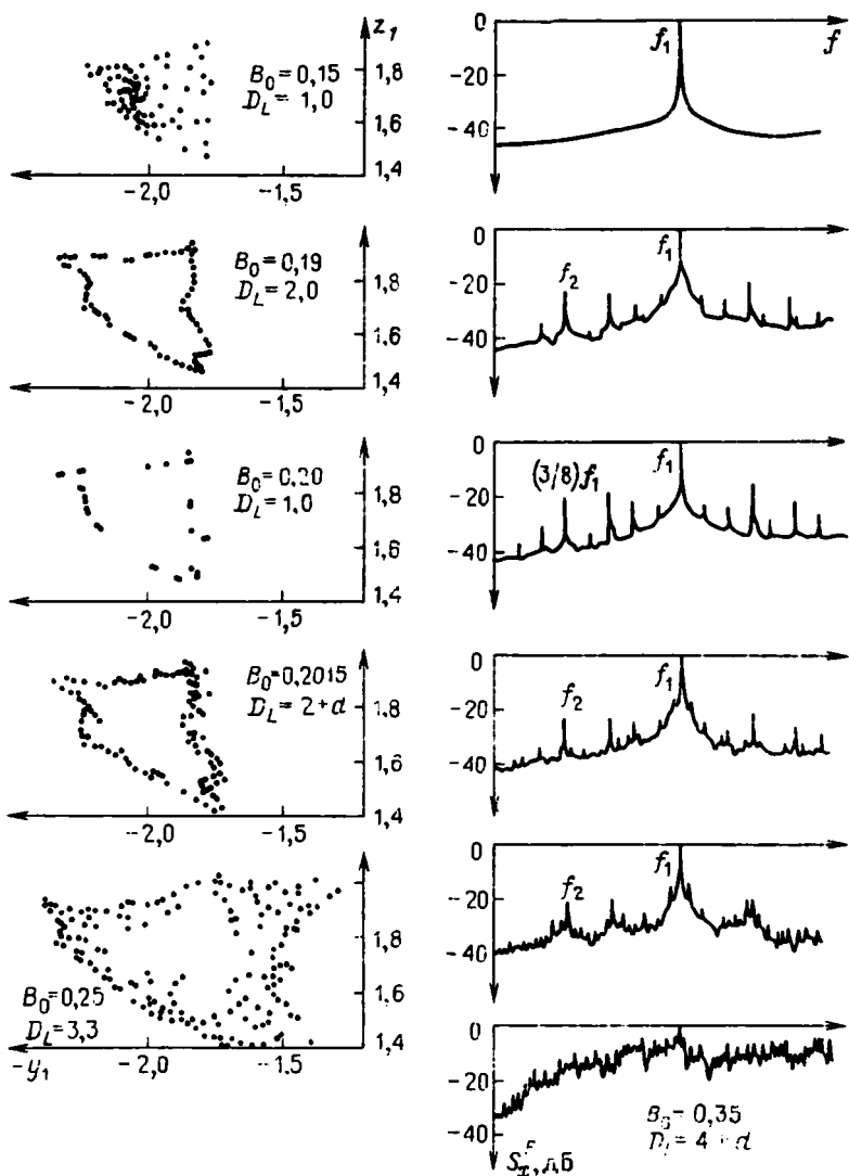
Р и с. 13.12. Проекция отображения Пуанкаре на плоскость -- y_1, z_1 (слева) и соответствующие спектры мощности колебаний (справа) с увеличением амплитуды внешнего воздействия на частоте f_{вн} = f_1
