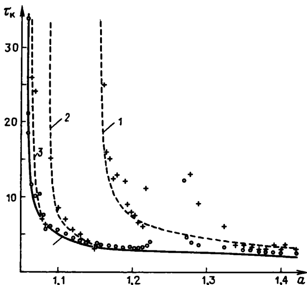
Р и с. 11.3. Зависимость времени корреляции \tau_k от параметра a отображения Хенона в отсутствие шума: 1 - a^* = 1,155 ; 2 - a^* = 1,088 ; 3 - a^* = 1,064
