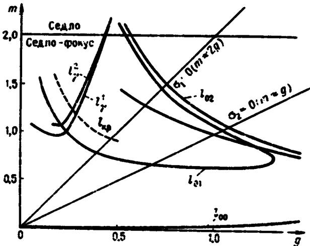
Р и с. 10.2. Бифуркационная диаграмма для системы (10.1)
