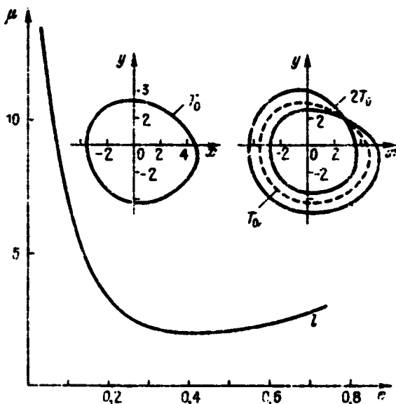
Р и с. 6.5. Бифуркационная линия удвоения периода циклов для системы Рёслера (6.29) на плоскости параметров e, \mu для b = 0,2
