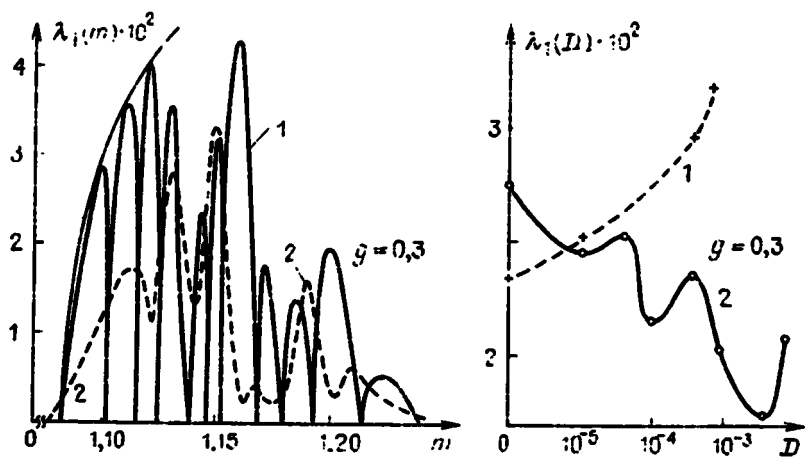
Р и с. 9.5. Влияние шумов на степень хаотичности движения: а - \lambda_1(m) для D = 0 (кривая 1) и D = 10^{-2} (кривая 2). б - \lambda_1(D) для m = 1,10050 (кривая 1), m = 1,10190 (кривая 2); m^* = 1,10112
