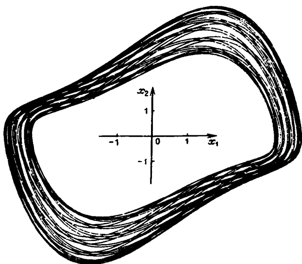
Р и с. 1.6. Проекция двумерного тора на плоскость переменных x_1 , x_2 . Численное интегрирование системы (1.25) проведено для значений параметров a = 1 ; b = 0,3 ; V = 1,0 ; \Gamma = 1,5 ; \varphi_0 = 0
