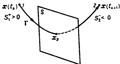
Р и с. 6.1. К иллюстрации метода расчета точки пересечения траектории с секущей поверхностью S
