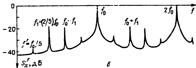
Р и с. 13.4. а – Бифуркационная диаграмма системы (13.1) вблизи резонанса 2/5 . б – Спектр мощности резонансного цикла \Gamma^+ на торе, рассчитанный для точки O
