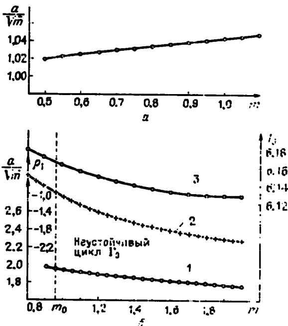
Р и с. 7.7. а - Зависимость нормированной амплитуды устойчивого цикла \Gamma_0 от параметра m . б - Зависимость амплитуды a/\sqrt{m} (1), мультипликатора \rho_1 (2) и периода T_0 (3) цикла \Gamma_0 от параметра m при прохождении точки бифуркации удвоения периода
