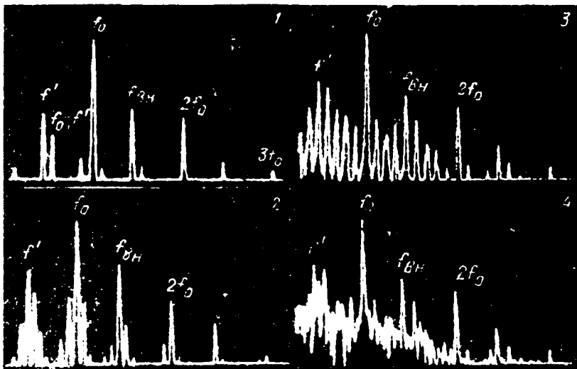
Рис. 12.9. Спектры мощности колебаний при движении по плоскости параметров (рис. 12.7) в направлении D : 1 - спектр гладкого тора, 2, 3 - развитие эффекта потери гладкости, 4 - спектр "тор — хаос" при малой надкритичности
