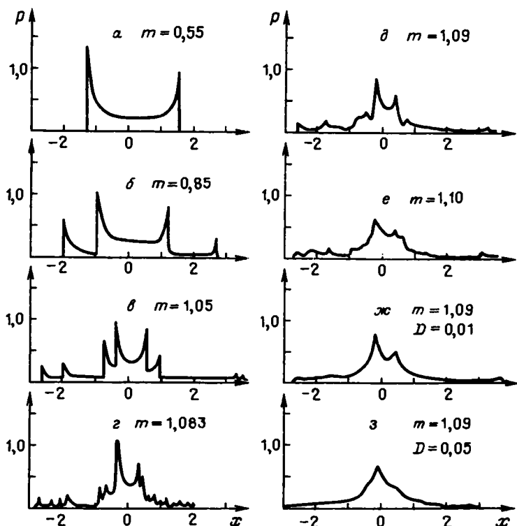
Р и с. 11.5. Эволюция одномерного распределения \rho(x) в системе (7.38) при вариации параметра m
