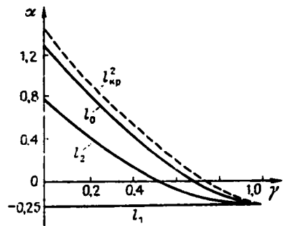
Р и с. 13.7. Бифуркационные линии l_{0,1,2} потери устойчивости неподвижными точками на плоскости параметров отображения (13.7); l_{кр} — линия разрушения инвариантных кривых L с рождением тор-аттрактора
