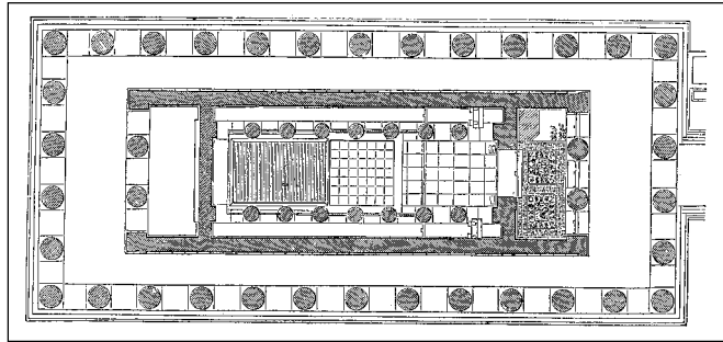
Рис. 317. План храма Зевса в Олимпии. По Дёрнфельду
