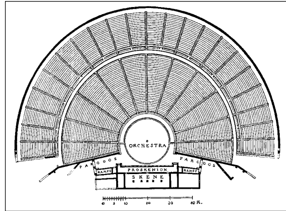
Рис. 386. План театра в Эпидавре. По Дёрнфельду и Рейшу
