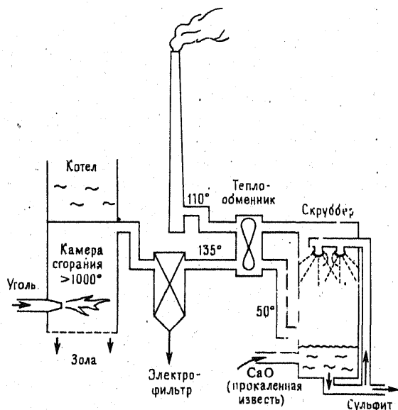
Рис. 2.12. Схема очистки топочных газов методом компании Кнауф Рисч Коттрелл.
