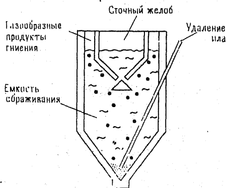
Рис. 3.6. Схема отстойника.
