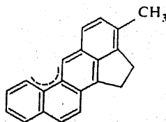
3-Метил- холантрен
