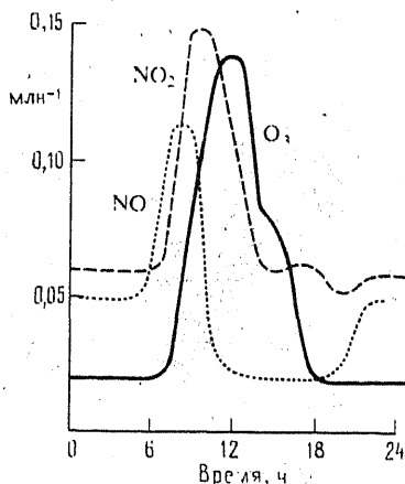
Рис. 2.9. Суточные изменения концентрации NO, NO 2 и O 3 в слоях атмосферы, близких к Земле [16].
