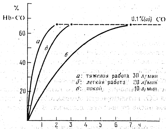
Рис. 2.8. Насыщение гемоглобина при различной физической нагрузке.
