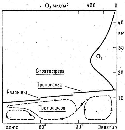
Рис. 2.2. Вертикальное строение атмосферы Земли.
