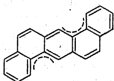
1,2-5,6-Дибенз- антрацен
