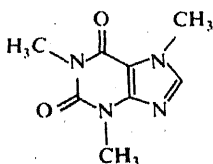
Кофеин
