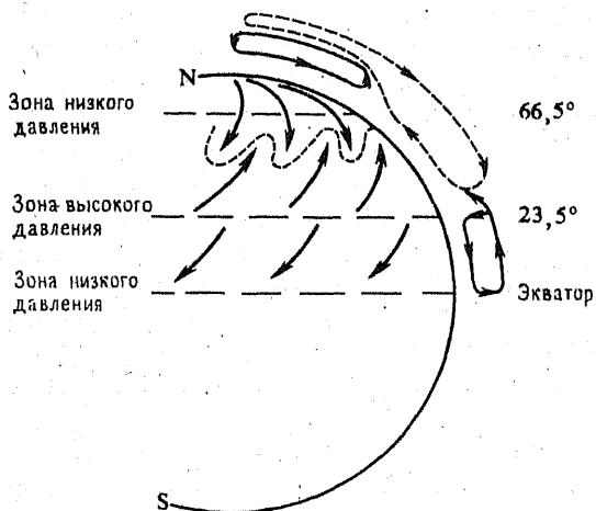
Рис. 2.1. Пояс ветров Земли.
