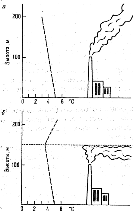
Рис. 2.7. Примеры распространения выбросов в атмосфере в зависимости от расположения ее тепловых слоев. a — нормальный градиент температуры (уменьшение с высотой); b — аномальный градиент температуры (увеличение с высотой).
