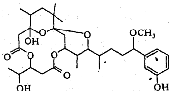
Дибромо-аплизиатоксин
