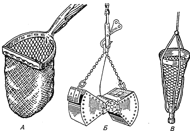
Рис. 33. Приспособления для взятия проб грунта и планктона:
